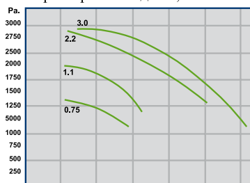
Характеристики для 7,5E- 15E
