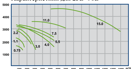
Характеристики для 25E- 90E
